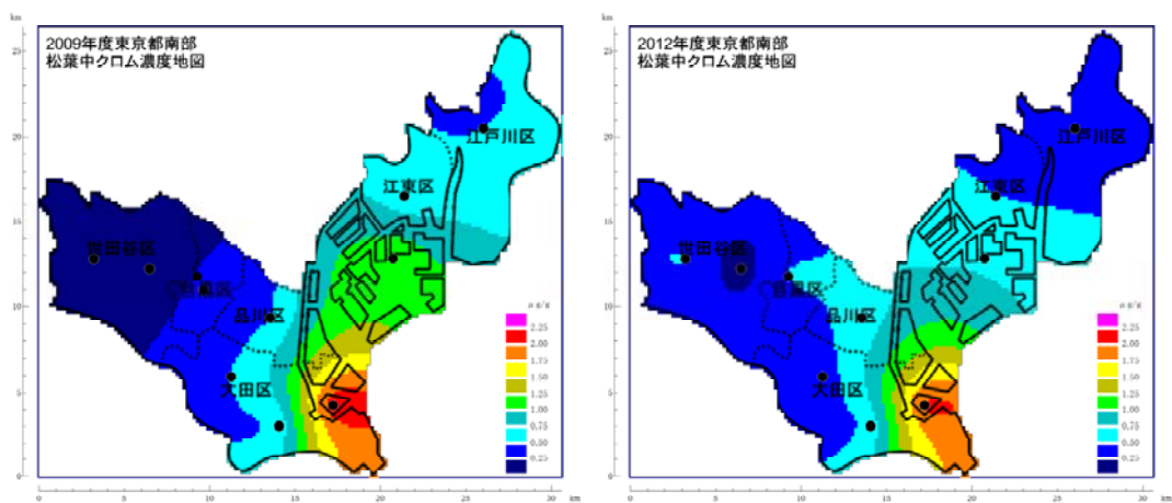
図 5 - 1 7 クロム
