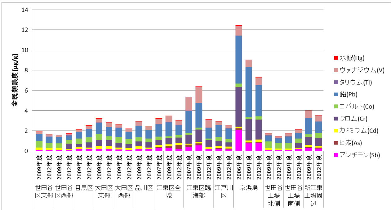
図5-1 マンガンと銅及びニッケルを除くその他の微量金属元素濃度の合計値比較
