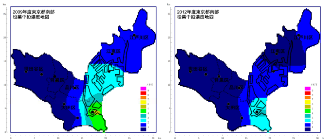
図5-20 鉛
