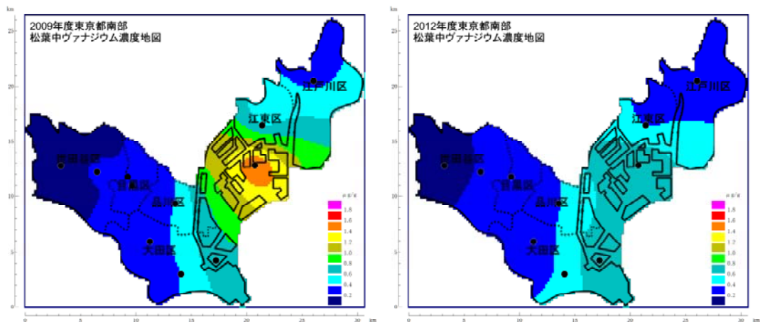
図5-24 ヴァナジウム
