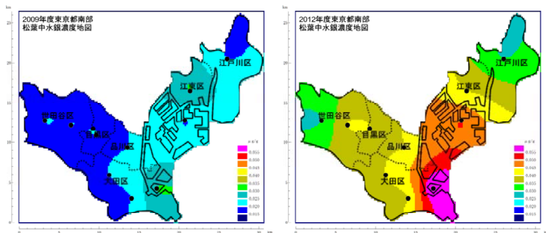
図5-25 水銀
