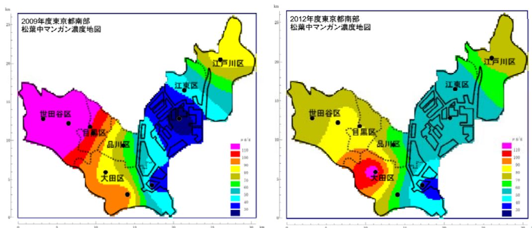
図5-21 マンガン
