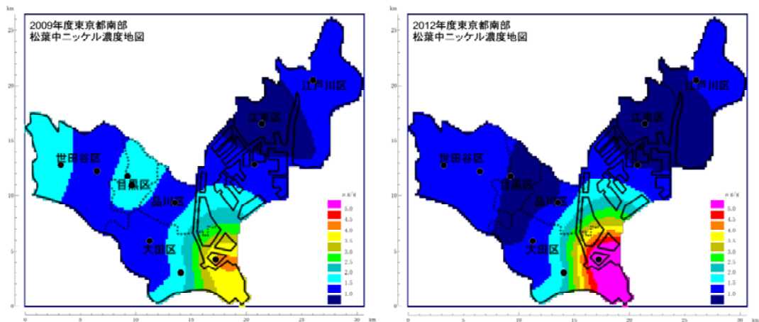
図5-22 ニッケル
