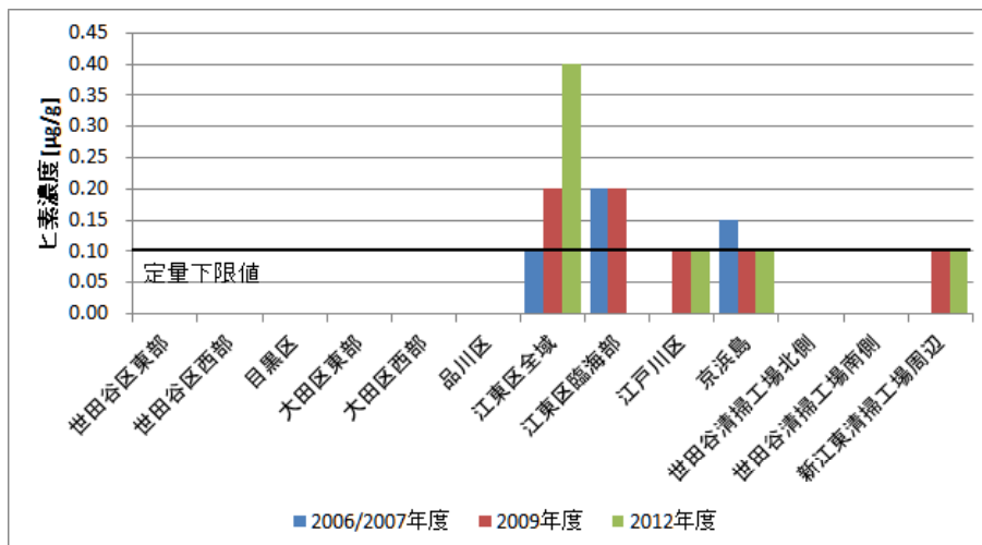
図5-3 ヒ素の濃度比較
