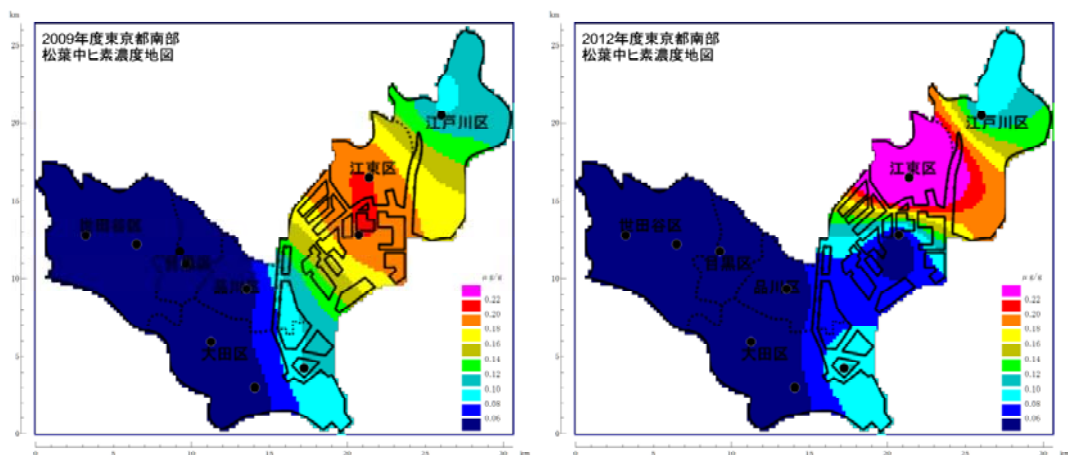
図5-15 ヒ素
