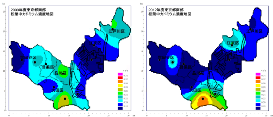
図 5 - 1 6 カドミウム
