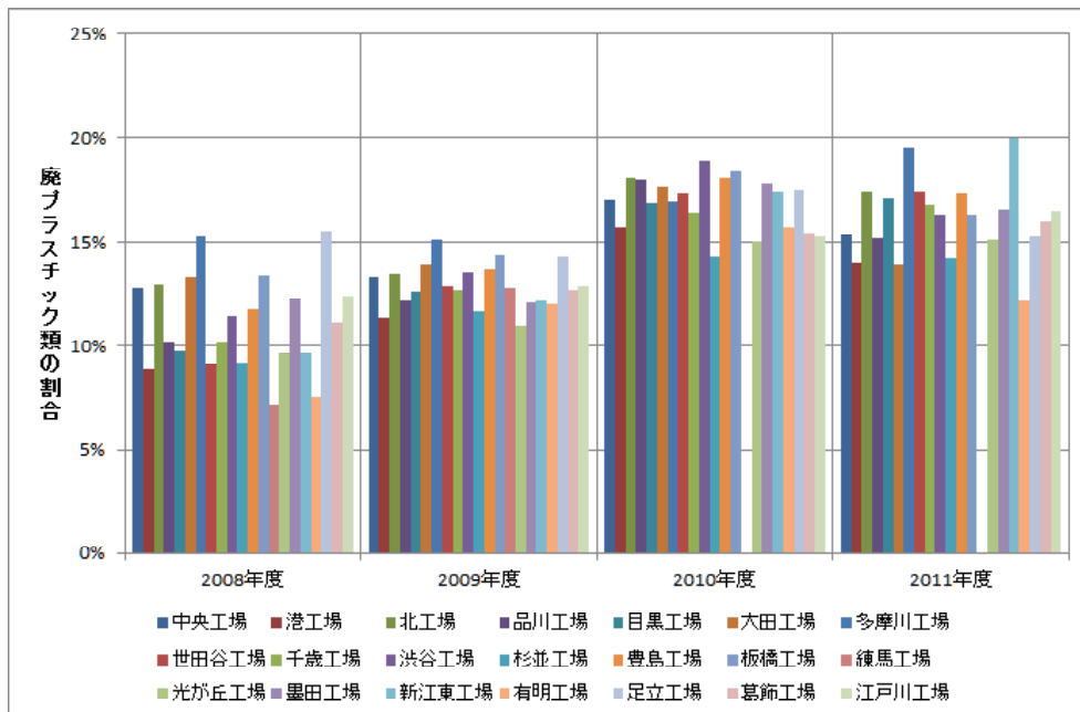
図 6-1 清掃工場に搬入されたごみに占める廃プラスチック類の割合
