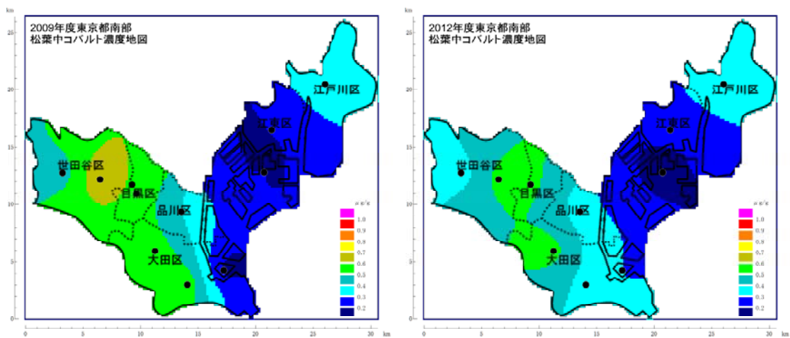
図 5 - 1 8 コバルト
