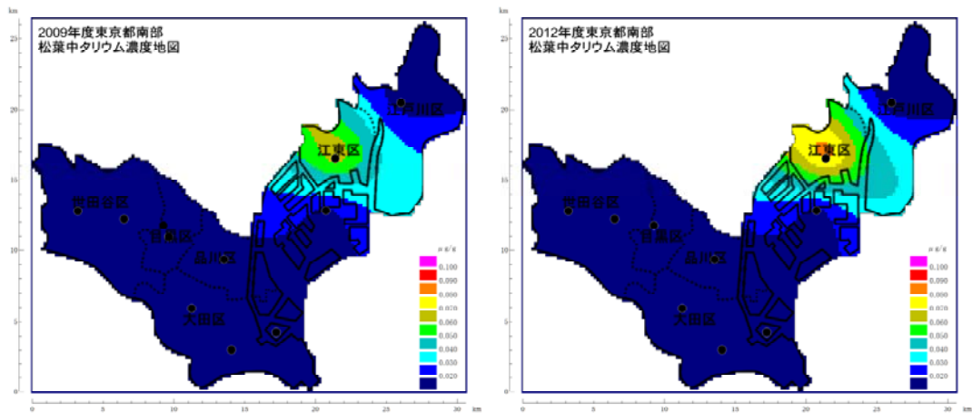
図5-23 タリウム
