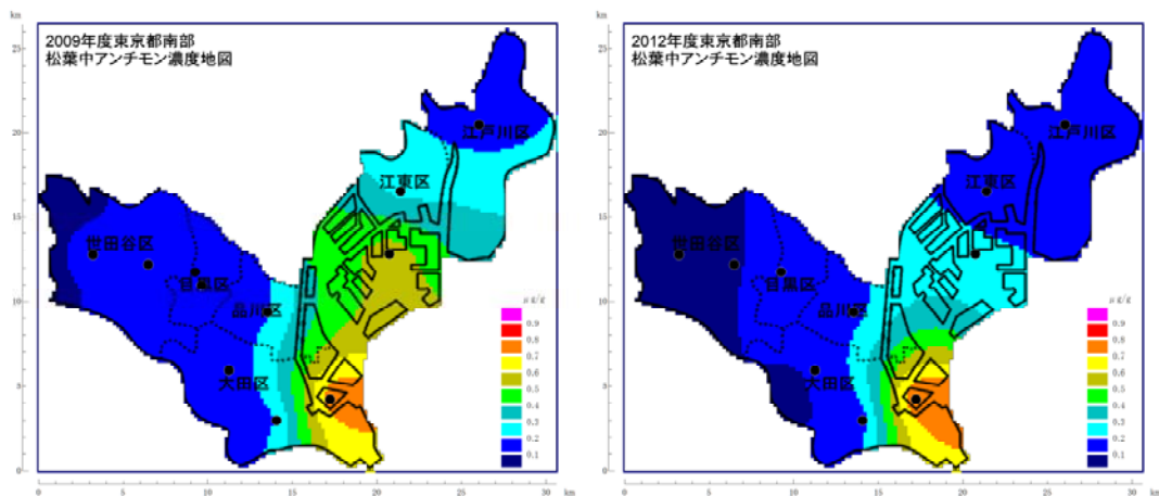
図5-14 アンチモン
